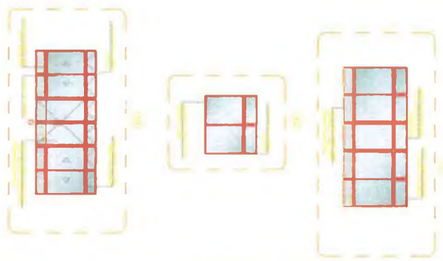
4 DETALHE Escala 1:50
