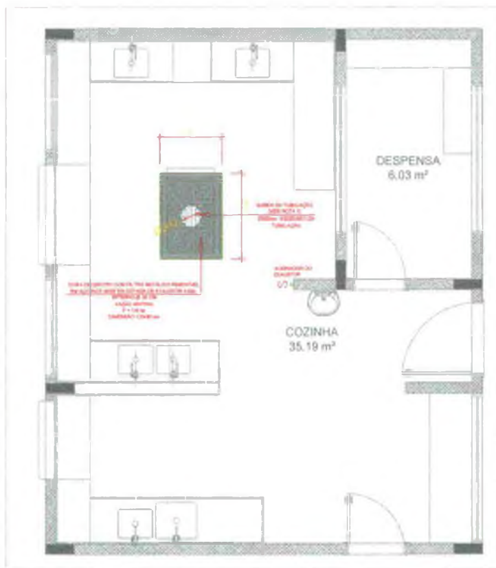
1 SISTEMA DE EXAUSTÃO - COZINHA BOTA-FLETA
