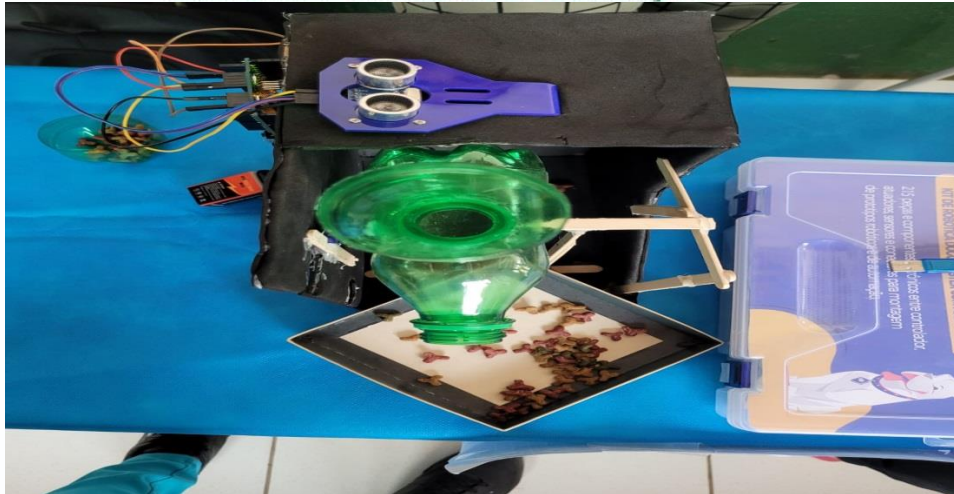
Figura 4: Dispensador de alimentos para animais com sensor de presença
